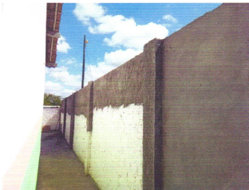
FOTO 03 - CHAPISCO APLICADO EM ALVENARIA (COM PRESENÇA DE VÃOS) E ESTRUTURAS DE CONCRETO DE FACHADA, COM COLHER DE PEDREIRO. ARGAMASSA TRAÇO 1:3 COM PREPARO EM BETONEIRA 400L. AF_10/2022
